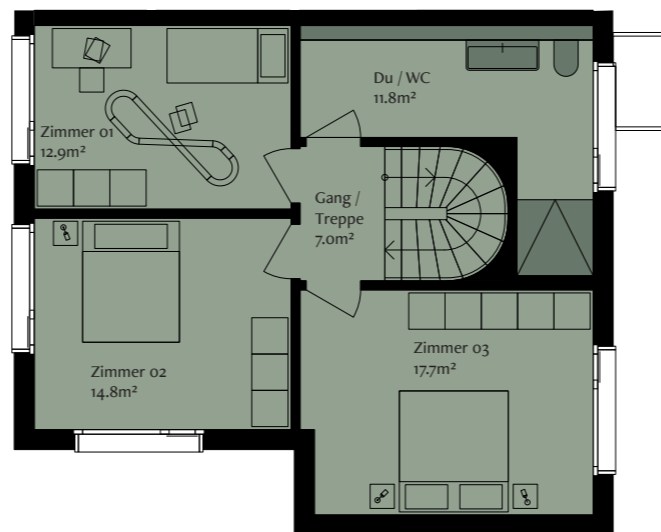
Obergeschoss
