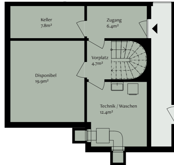
Untergeschoss
