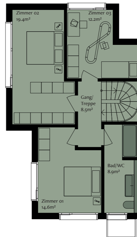
Obergeschoss
