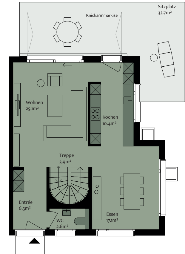
Erdgeschoss
