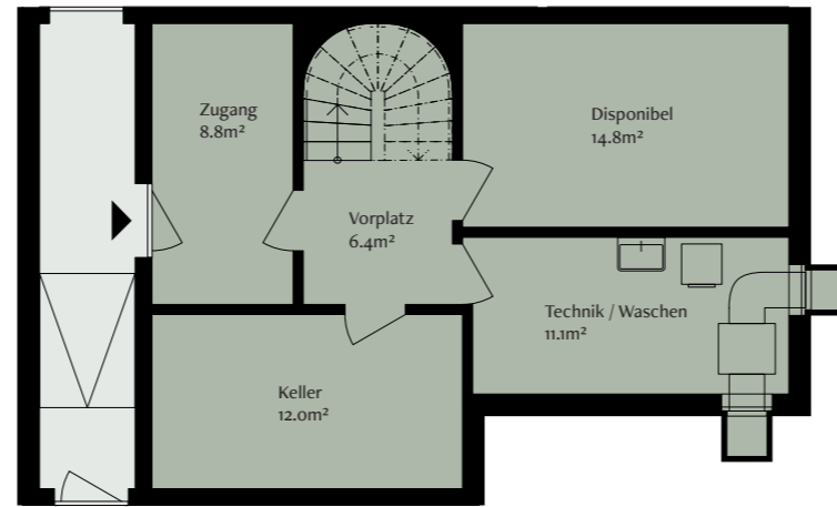
Untergeschoss
