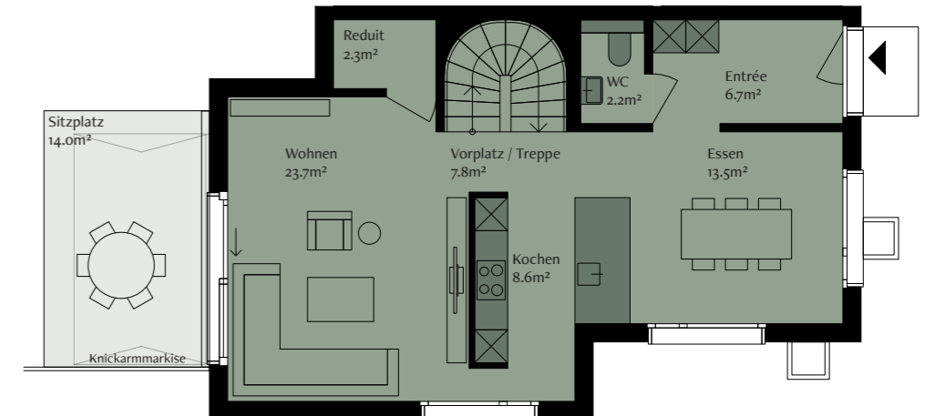
Erdgeschoss
